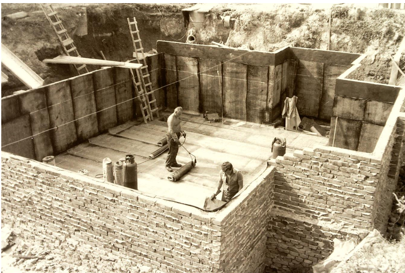
Budování základů nové přístavby v roce 1979.
