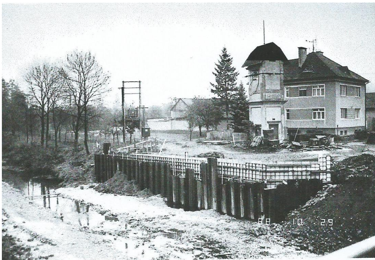
Zahájení výstavby nového mostu v roce 1988.
